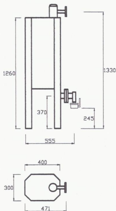
Šema isparivača 100 kg/h
