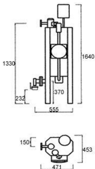
Šema isparivača 50 kg/h
